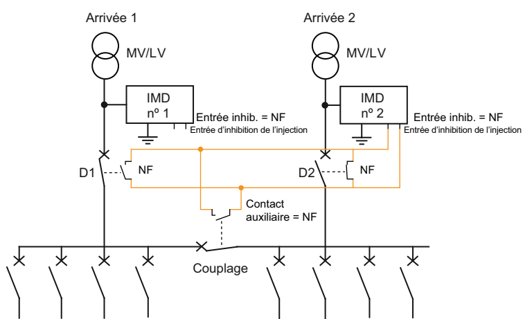
Utilisation de disjoncteurs avec contacts auxiliaires normalement fermés (NF) :
