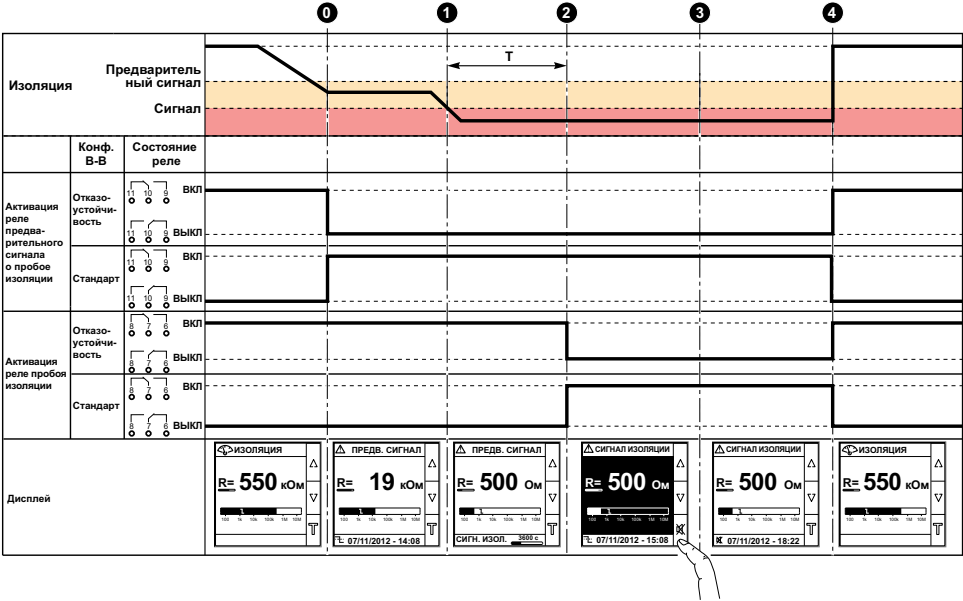
Реле подтверждения сигнала ВЫКЛ
