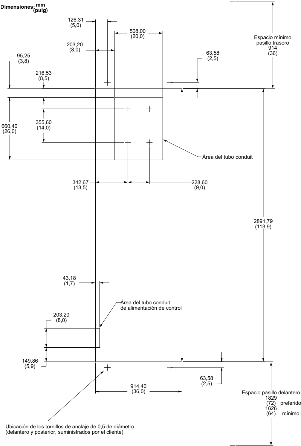
Figura 3 - Plano típico de planta: Unidad estándar de 914 mm (36 pulg) de ancho (no para la construcción)
