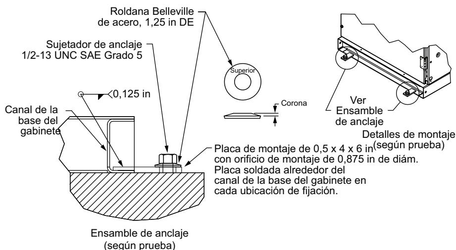
Figura 12 - Tablero de fuerza como ensamble de anclaje probado
