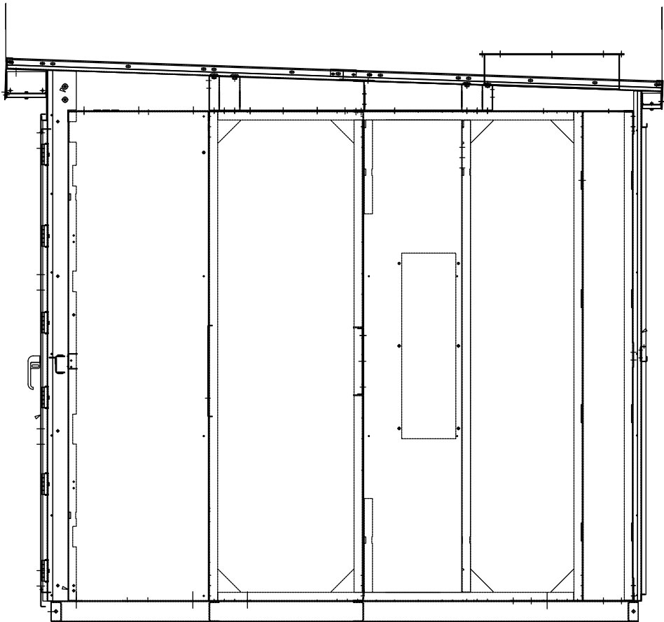
Figura 13 - Vistas frontal y lateral típicas: Tablero de fuerza sin pasillo de servicio
