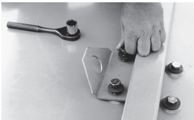
Figura 9 - Extracción de las orejas de izaje pequeñas
