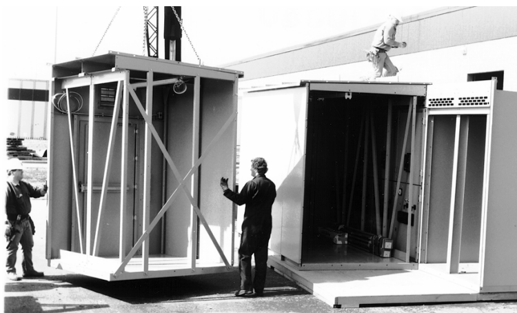
Figure 15 - Déplacement des sections avec des renforts en place
