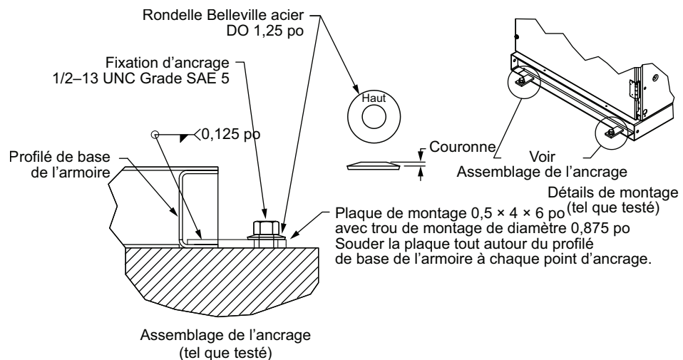
Figure 28 - Assemblage d'ancrage pour appareillage de commutation tel que testé
