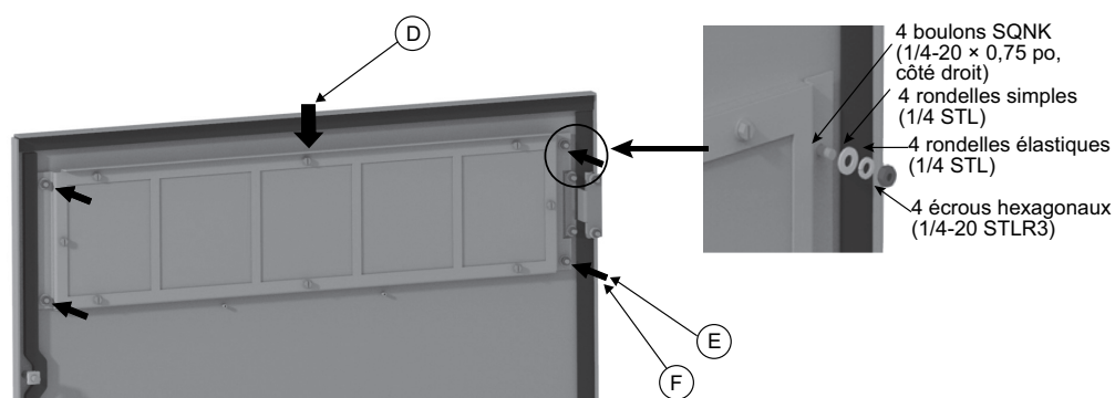
Figure 38 - Réinstallation du nouveau filtre (volet supérieur)
