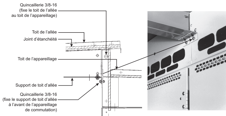
Figure 13 - Ancrage du support de toit d'allée sur l'appareillage de commutation
