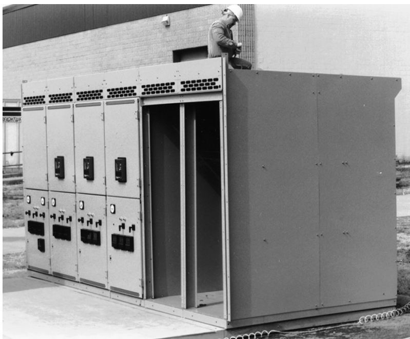
Figure 10 - Sécurisation d'un espace pour équipement pour l'appareillage de commutation
