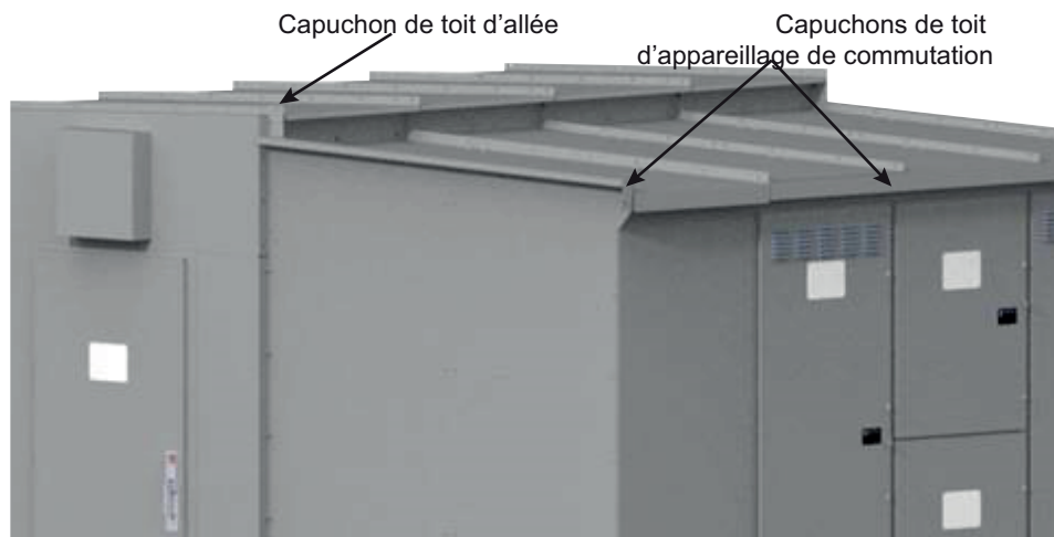
Figure 20 - Montages des capuchons de toit
