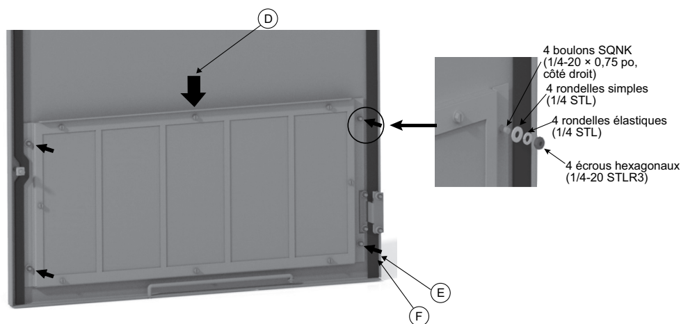
Figure 35 - Réinstallation du nouveau filtre (volet inférieur)
