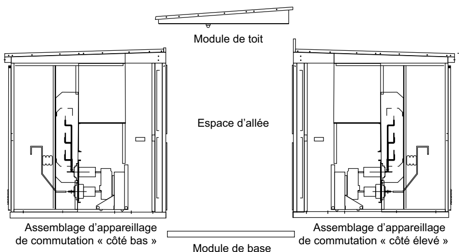
Figure 26 - Configuration d'une allée commune
