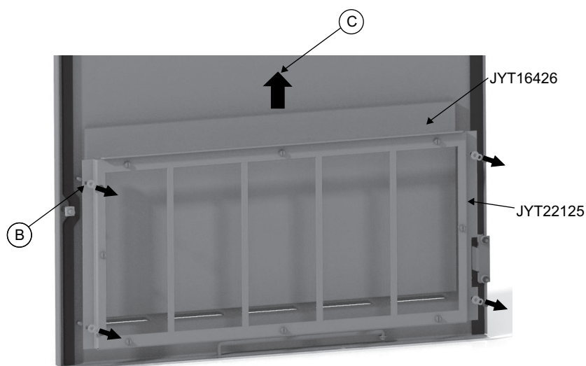
Figure 34 - Retrait du filtre usagé (volet inférieur)
