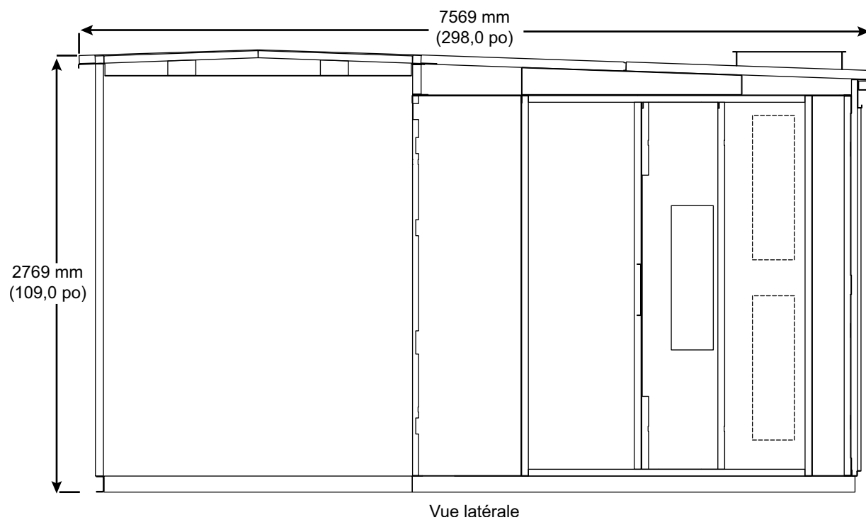
Figure 39 - Plan d'encombrement d'une armoire à allée unique
