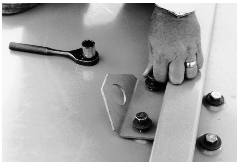
Figure 23 - Retrait des petites pattes de levage
