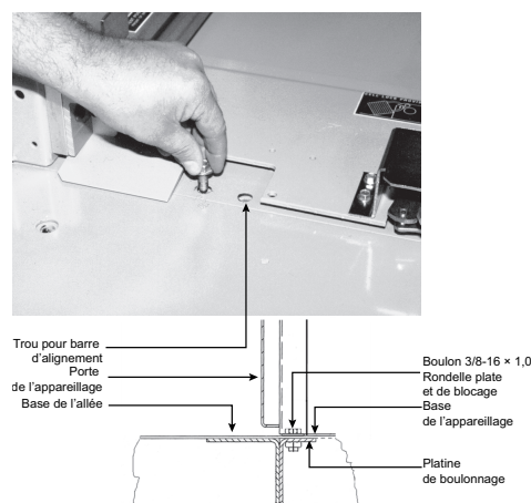
Figure 14 - Connexion de la base de l'allée et de l'appareillage de commutation
