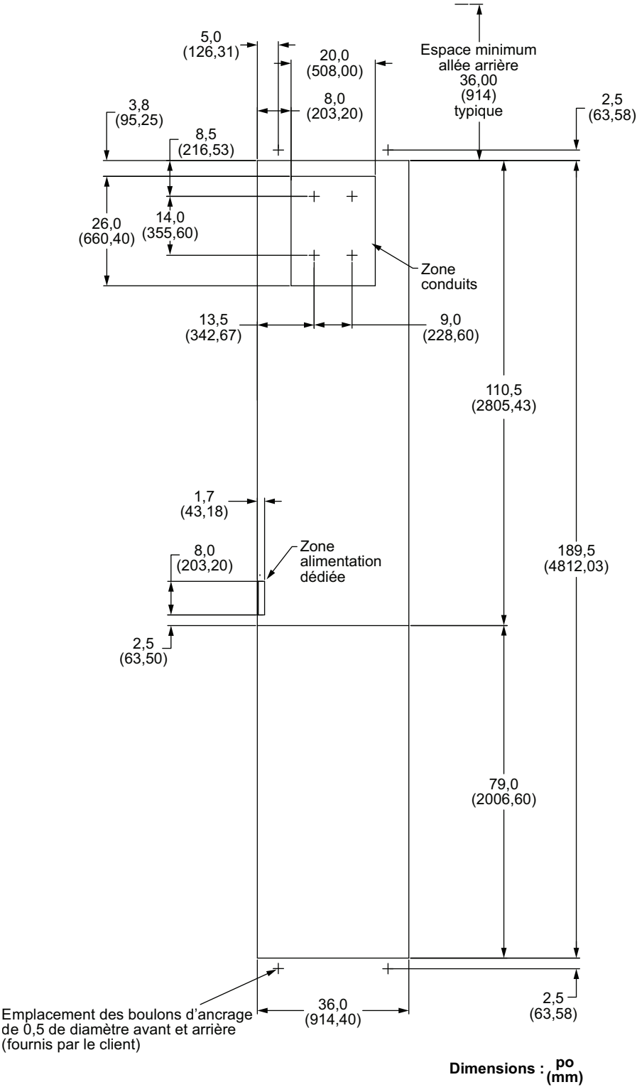
Figure 3 - Plan de sol à allée unique : Unité de 914 mm (36 po) de large standard (ne pas utiliser pour la construction)
