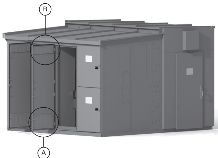
Figure 36 - Unités avec allée avec portes arrière ouvertes
