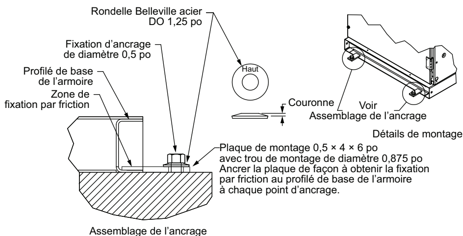
Figure 27 - Assemblage de l'ancrage pour appareillage de commutation non sismique
