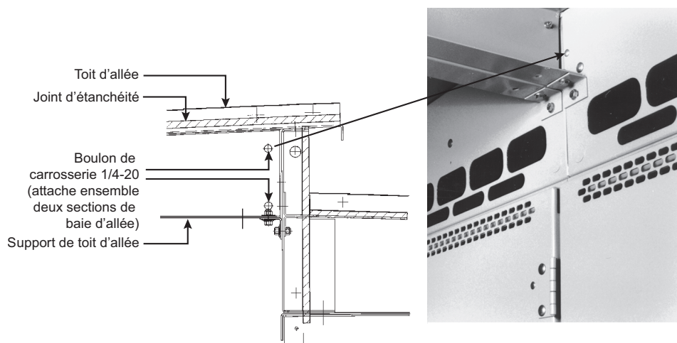
Figure 18 - Attachement de la deuxième section d'allée à la première section d'allée
