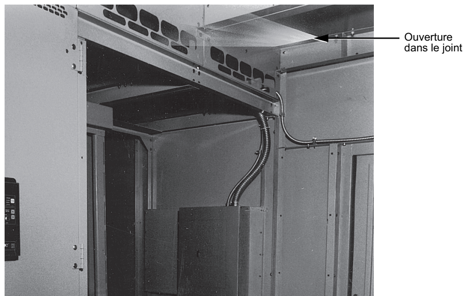
Figure 21 - Inspection du joint d'étanchéité de l'armoire
