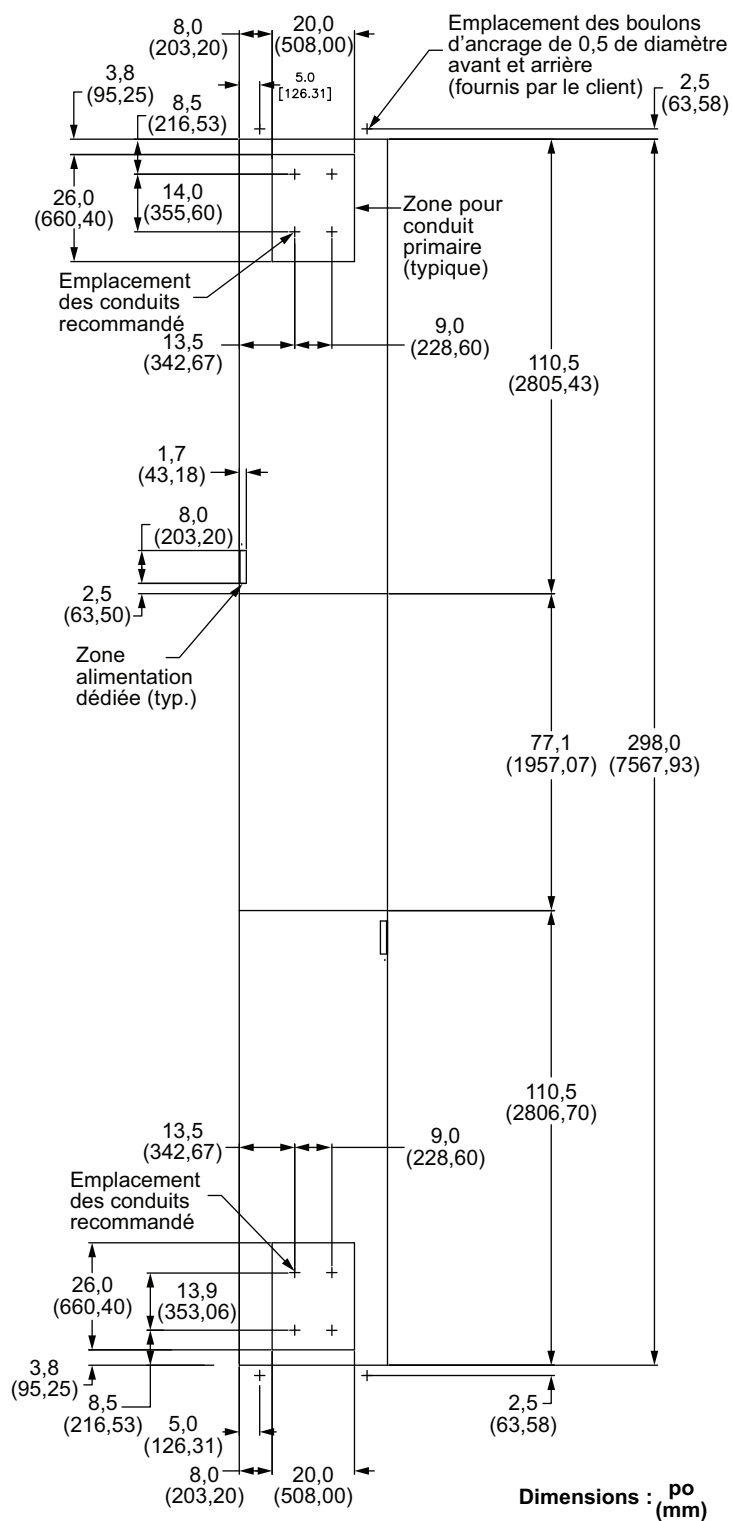
Figure 4 - Plan de sol à allée commune : Unité de 914 mm (36 po) de large standard (ne pas utiliser pour la construction)
