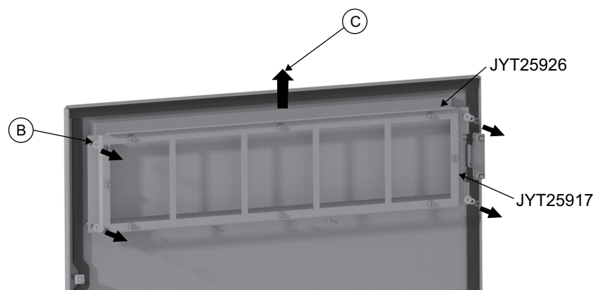
Figure 37 - Retrait du filtre usagé (volet supérieur)
