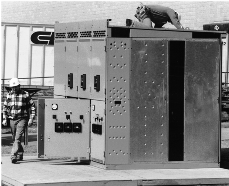
Figure 9 - Sécurisation des sections d'appareillage de commutation
