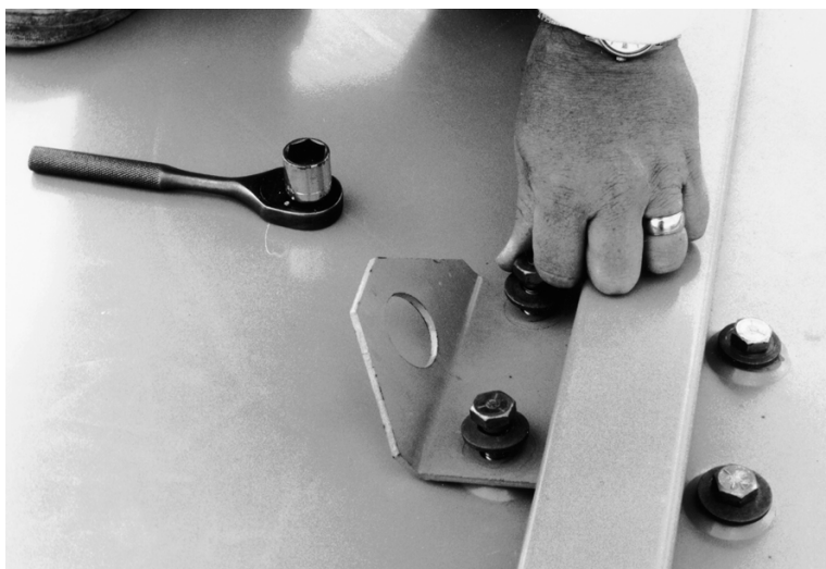
Figura 23 - Extracción de las orejas de izaje pequeñas
