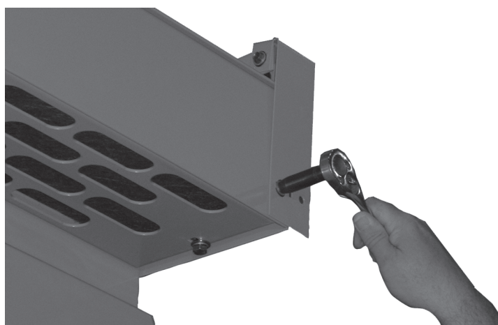
Figura 19 - Instalación de las tapas del techo
