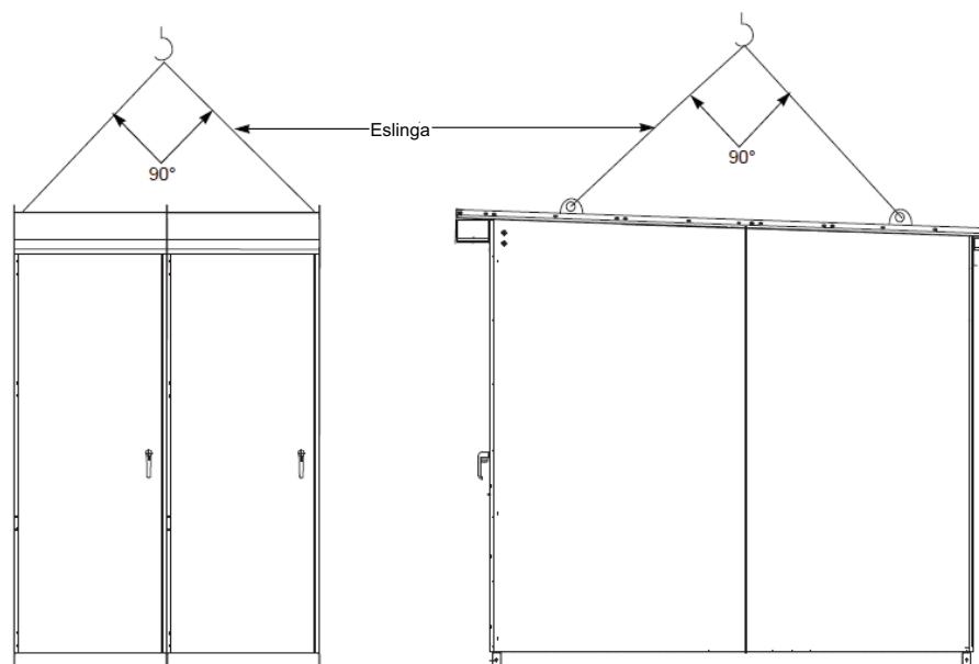
Figura 2 - Método de izaje
