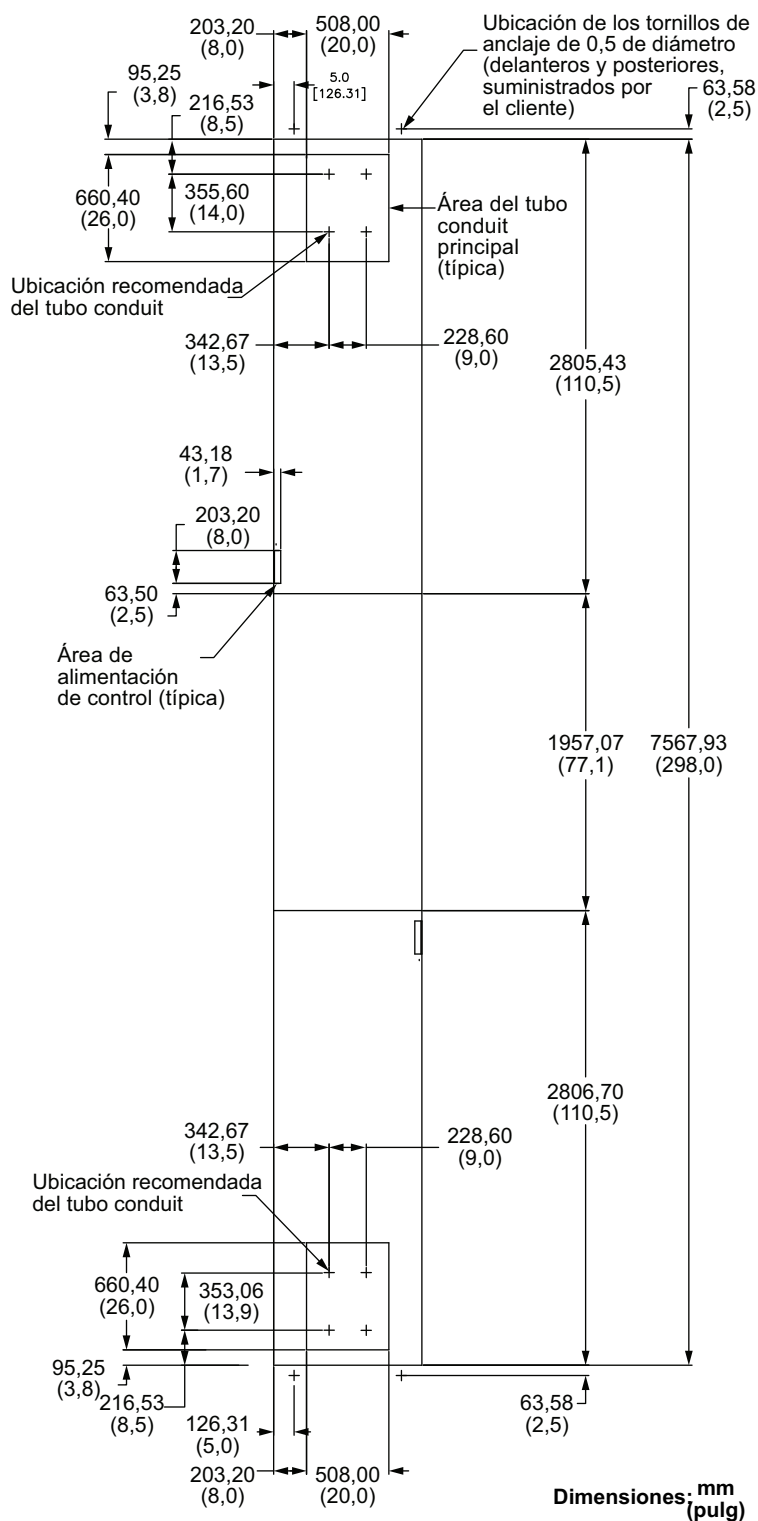
Figura 4 - Plano de planta del pasillo común: Unidad estándar de 914 mm (36 pulg) de ancho (no para la construcción)
