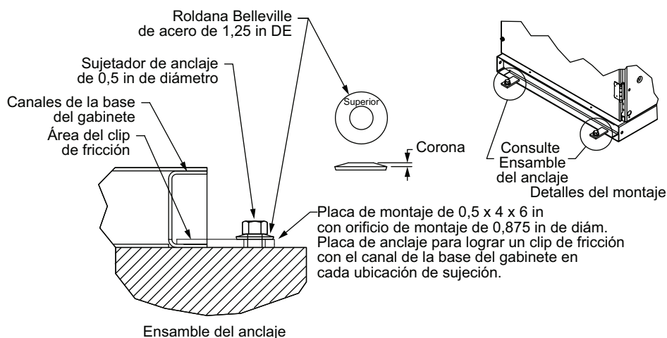
Figura 27 - Conjunto de anclaje del tablero de fuerza no sísmico
