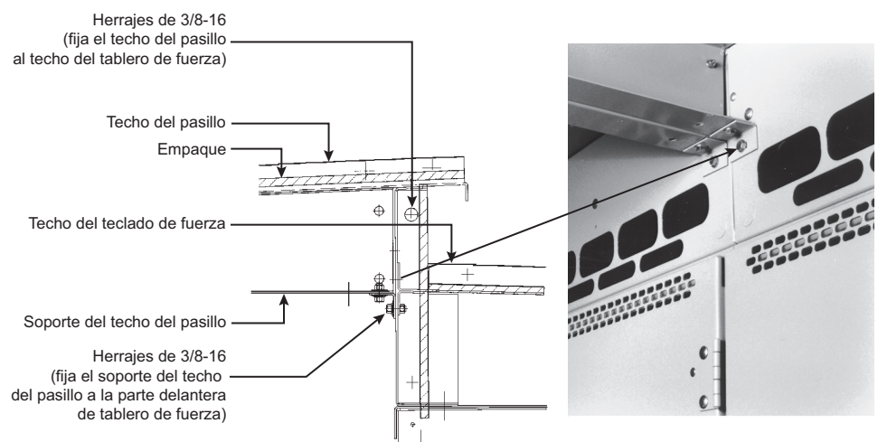
Figura 13 - Anclaje del soporte del techo del pasillo al equipo del tablero de fuerza
