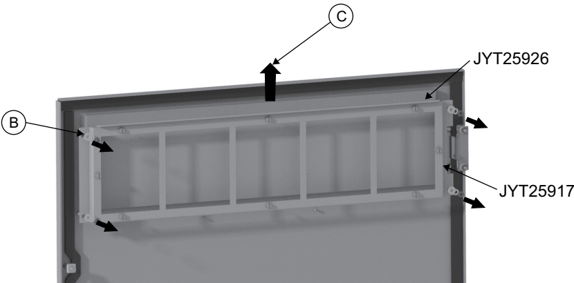
Figura 38 - Sustitución del nuevo filtro (rejilla superior)
