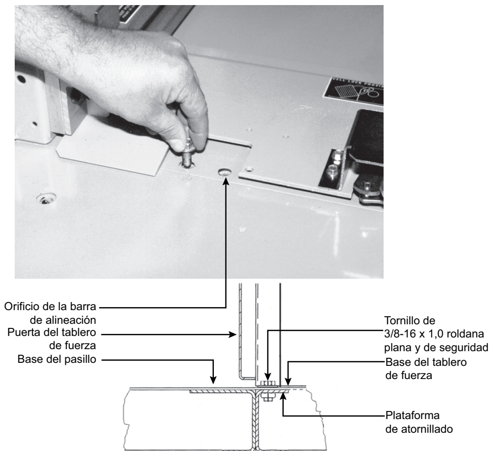
Figura 14 - Conexión de la base del pasillo y del tablero de fuerza
