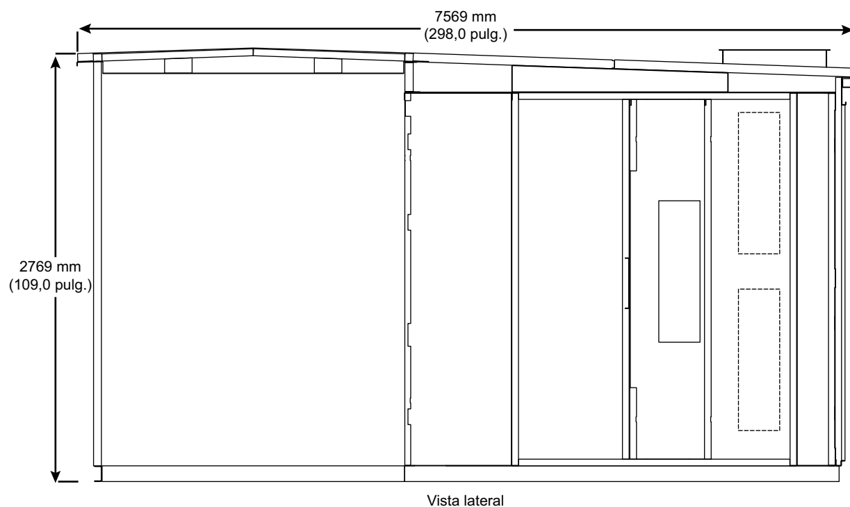
Figura 39 - Esquema de unidad con un solo pasillo de servicio
