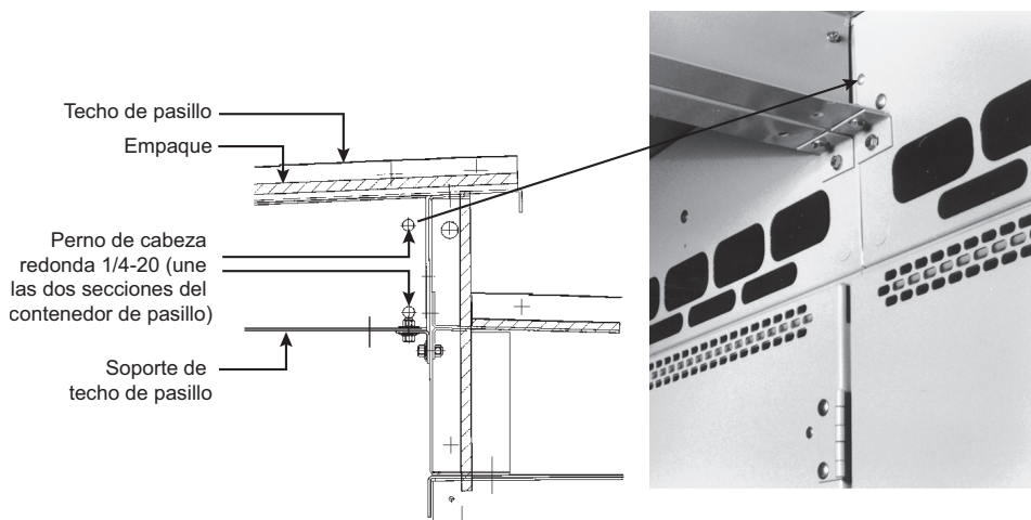
Figura 18 - Fijación de la segunda sección del pasillo a la primera sección
