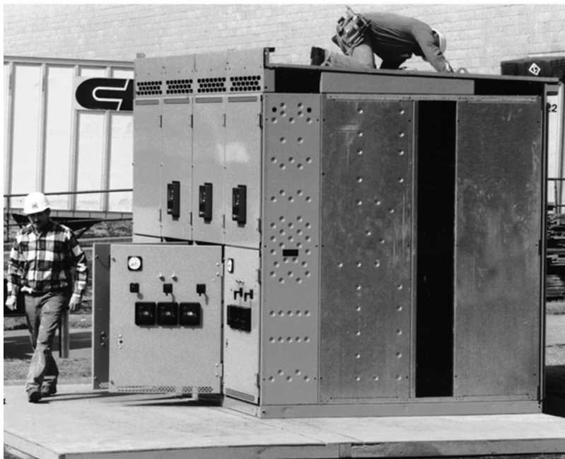
Figura 9 - Fijación de las secciones del tablero de fuerza
