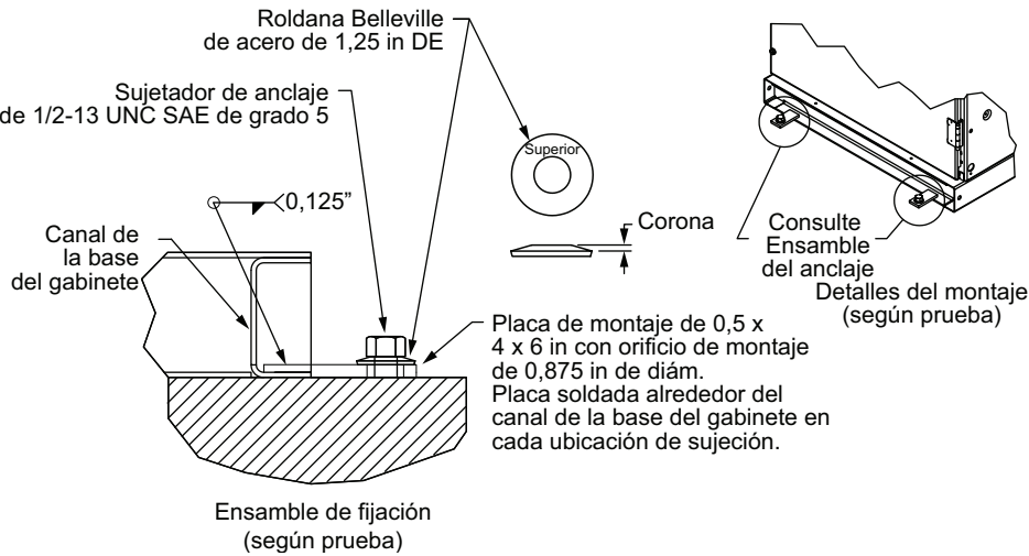
Figura 28 - Tablero de fuerza como ensamble de anclaje probado
