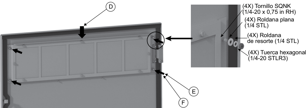
Figura 38 - Sustitución del nuevo filtro (rejilla superior)
