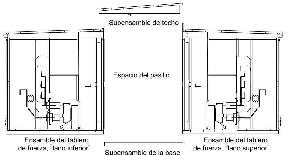
Figura 26 - Configuración del pasillo común
