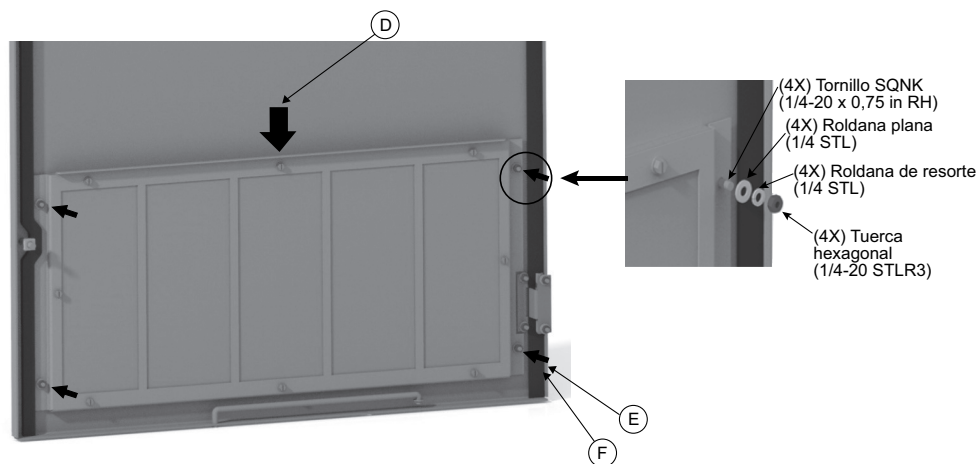
Figura 35 - Sustitución del nuevo filtro (rejilla inferior)
