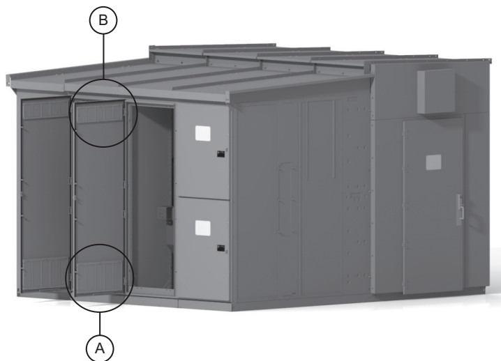
Figura 36 - Unidades con pasillo de servicio con puertas traseras abiertas
