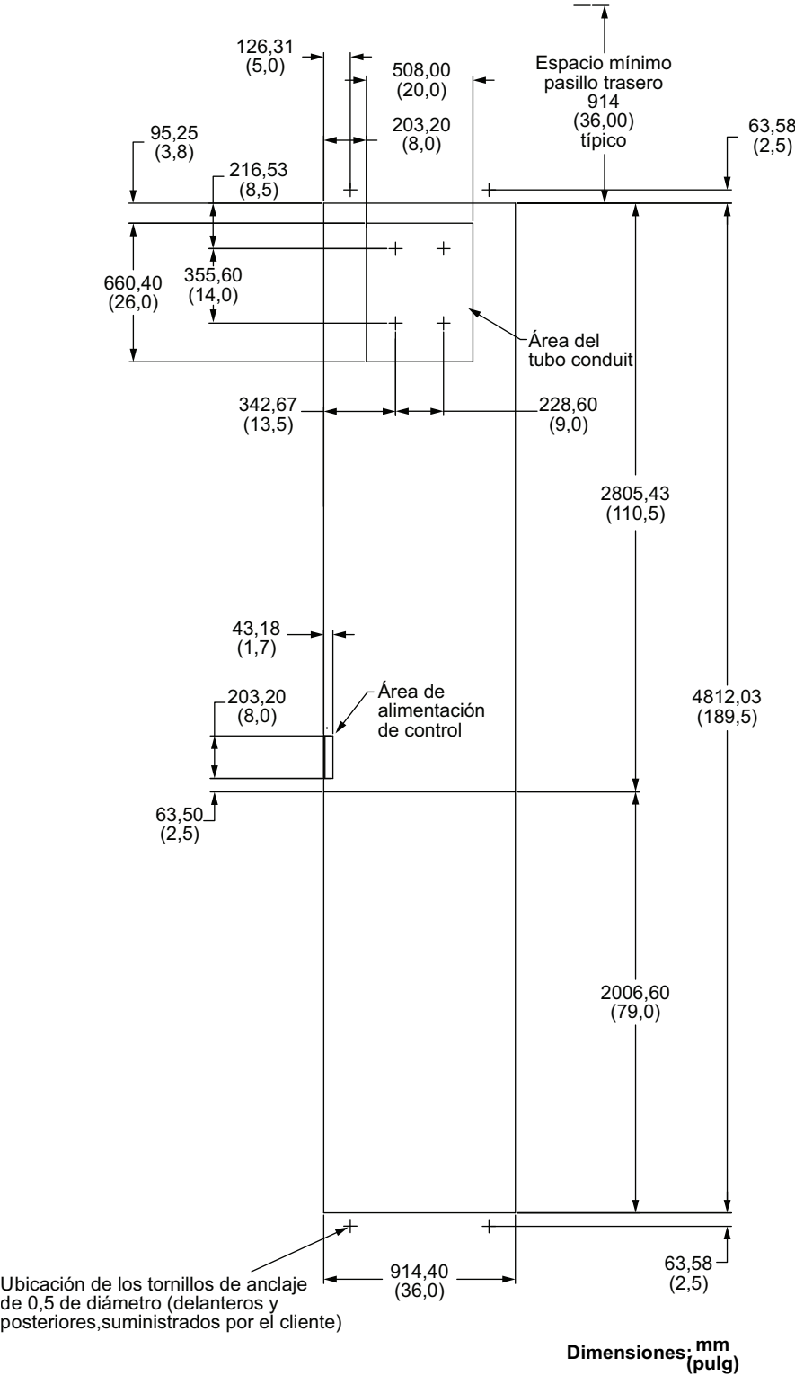
Figura 3 - Plano de planta de un solo pasillo: Unidad estándar de 914 mm (36 pulg) de ancho (no para la construcción)
