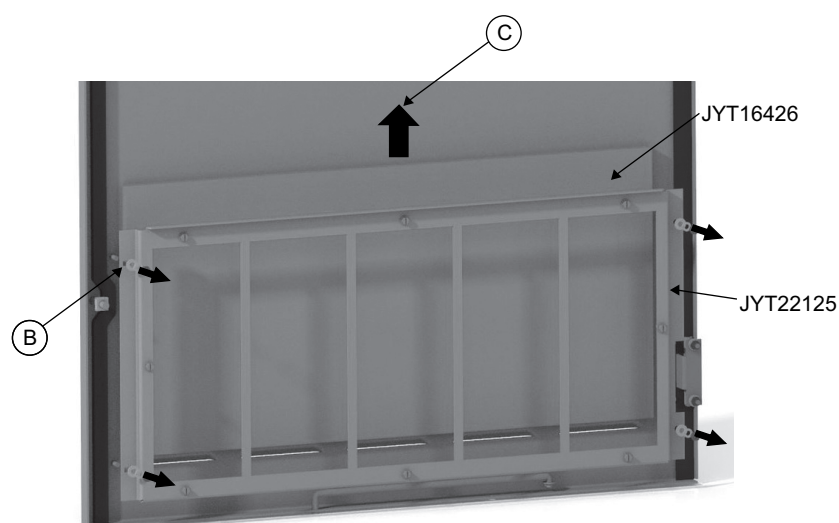
Figura 34 - Extracción del filtro usado (rejilla inferior)
