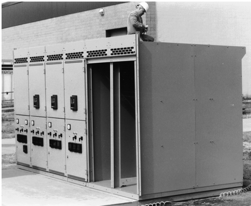
Figura 10 - Fijación de las secciones vacías para equipos al tablero de fuerza
