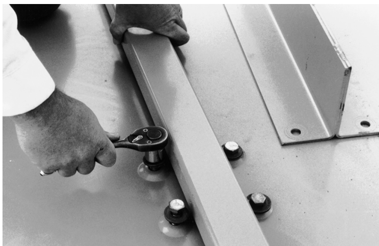
Figura 24 - Cómo tapar los orificios con pernos y arandelas de sellado
