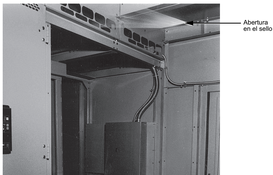
Figura 21 - Inspección del gabinete para descartar la presencia de aberturas en el sellado
