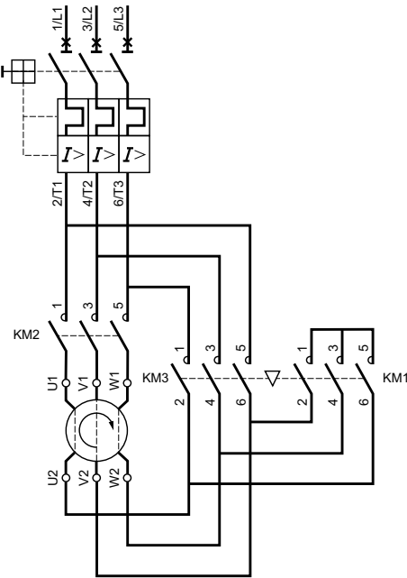
带热磁断路器和接触器的星三角电机启动器
