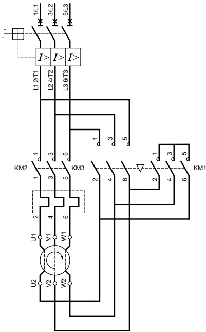
带热磁断路器、过载继电器和接触器的星三角电机启动器
